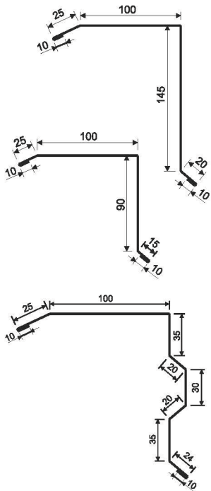
Вітрозахист 4/1
