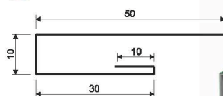
Планка для підшивки 12/1
