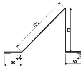
Трубчастий снігозатримувач універсальний L - 1500мм
