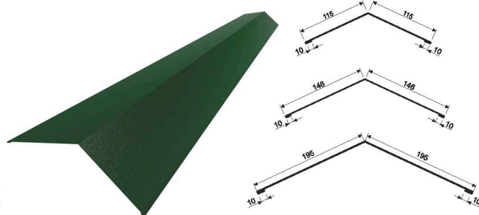
Трикутний 5/1
