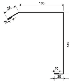
Для підшивки 4/1
