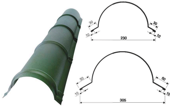
Універсальний 4/1
