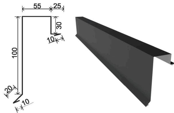
Планка з'єднання для фальца 20/1 - 2м 80/1 - 0.48м
