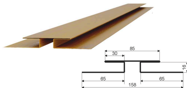
З'єднувальна планка 4/1
