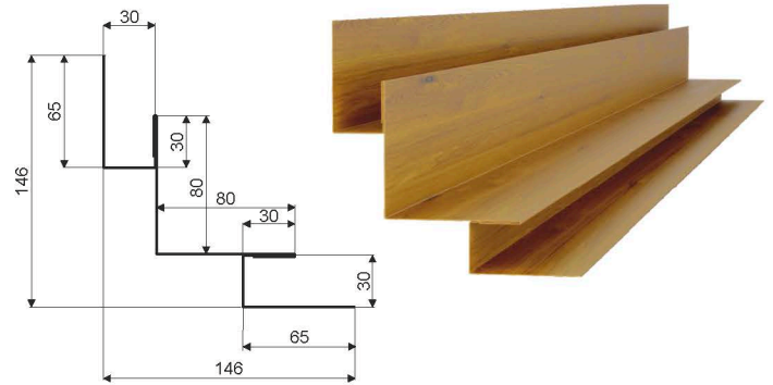
Кут внутрішній 2/1
