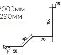
Стінний захист 4/1
