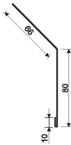
Захист карниза 8/1
