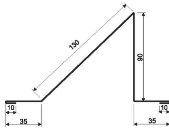
Великий 6/1
