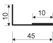
Г-планка 19/1
