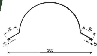
Універсальний 3/1
