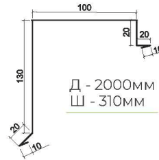
Вітрозахист 4/1
