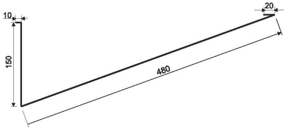
Закоминева планка 3/1
