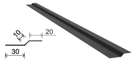
Планка з'єднання для фальца 20/1 - 2м 80/1 - 0.48м
