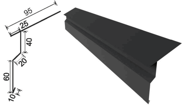
Вітрозахист для фальца 5/1
