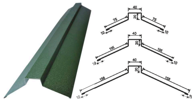
Декоративний 4/1
