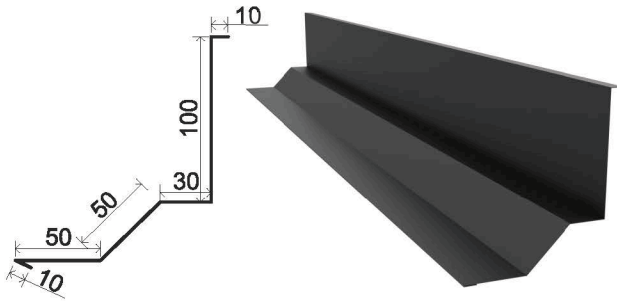
Стінний захист для фальца 5/1
