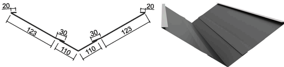
Жолоб плоский 2/1
