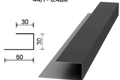
П-планка для фальца 11/1 - 2м 44/1 - 0.48м
