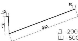
Закоминава планка 2/1
