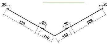
Коньок декоративний 4/1
